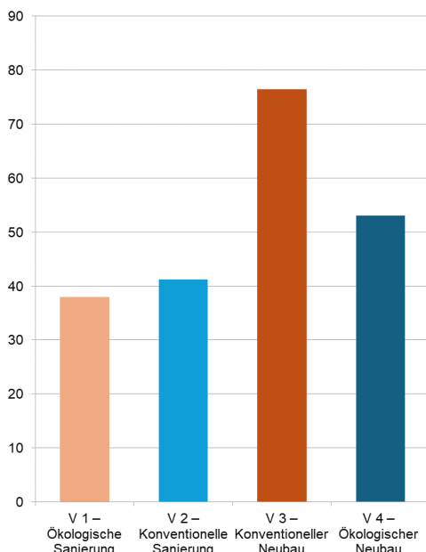
Bilanz eines Beispielobjekts Global Warming Potential, total [kg CO 2 -Äqv./ m 2 NGFa]
